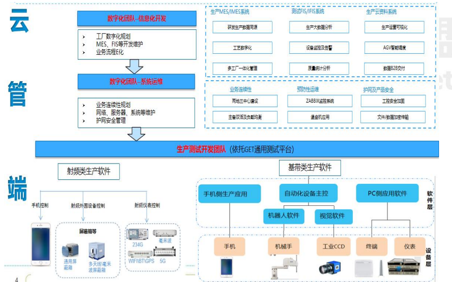
图 4 中兴终端制造基于“云管端”的云测试综合方案设计模型
