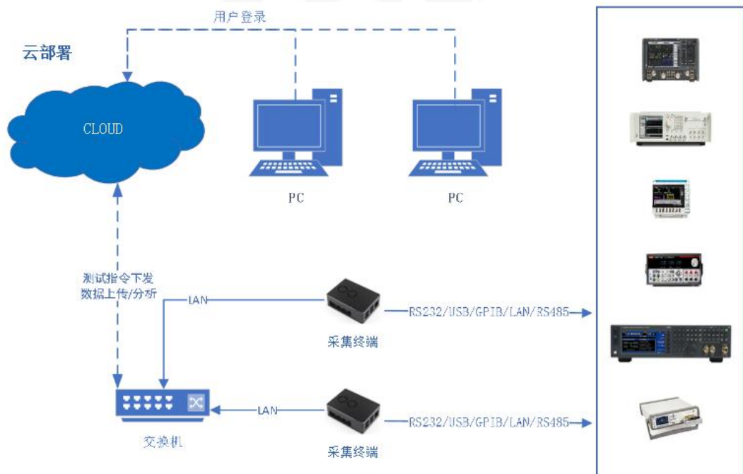
图 10 生产云测试架构（部分传输已经升级为光纤通信方案）
