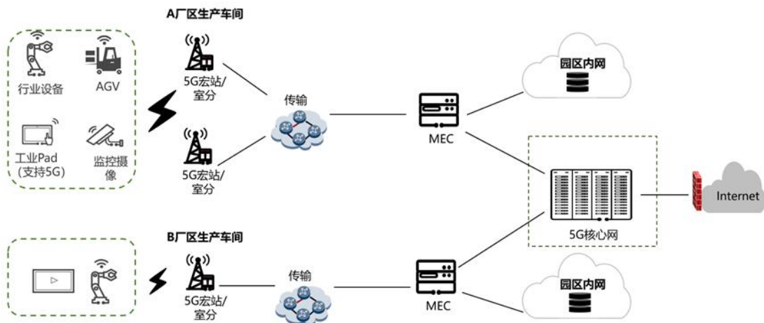
图 4-5 跨园区 5G 专网部署
