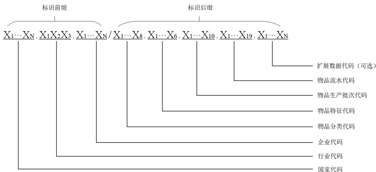
图 1 航天行业物品标识编码结构
