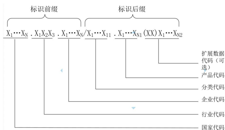
图1 燃气设备材料标识编码结构
