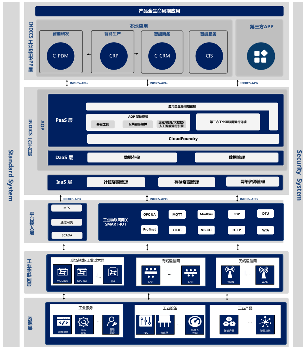
INDICS 平台架构图
